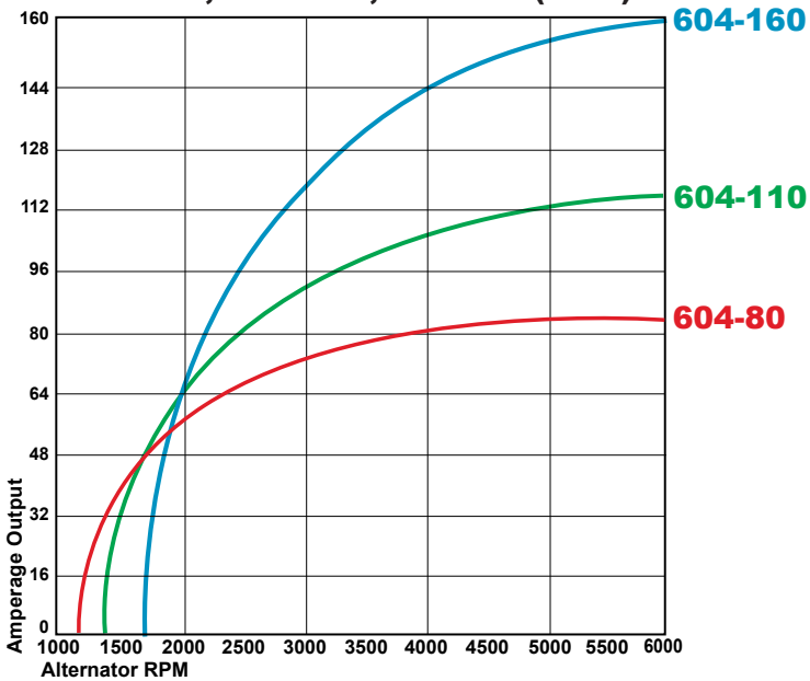
BALMAR Curve Comparison 604-80, 604-110 , 604-160 (& IG)
